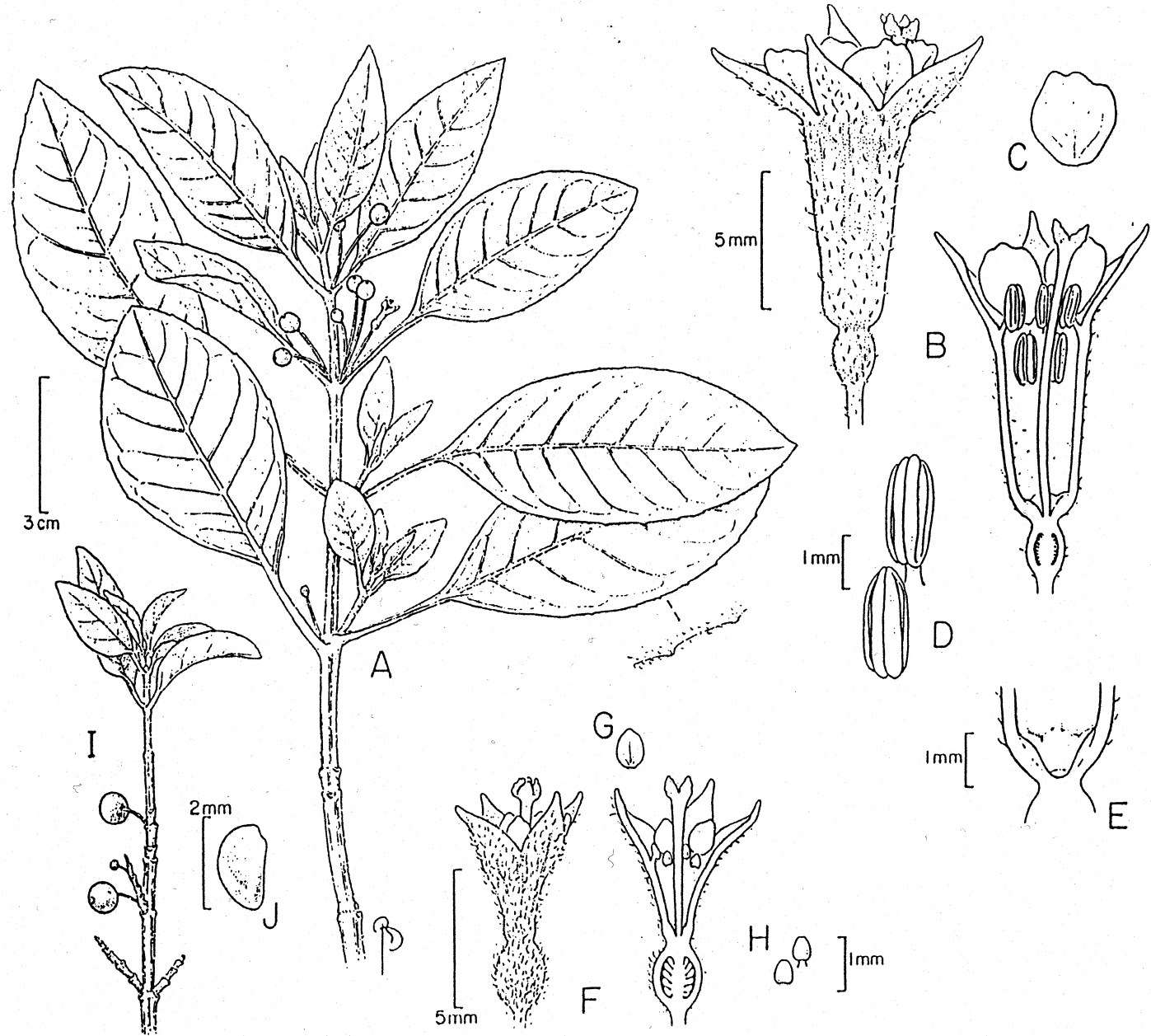
Fuchsia ravenii
